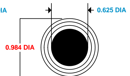
3/4" MINI Tri-Clamp
