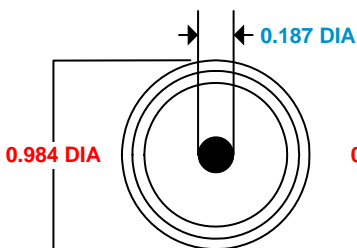
1/4" MINI Tri-Clamp
